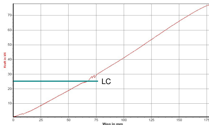
Bild 17: Last/Dehnungs-Diagramm eines 50 mm Polyester Gurts (Quelle: Dolezych)
