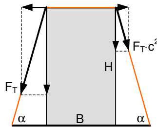
Bild 6: Komponenten einer Niederzurrung mit unterschiedlicher Vorspannung
