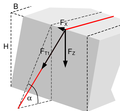
Bild 19: Sicherungswirkung durch Kräfte längs zum Fahrzeug
