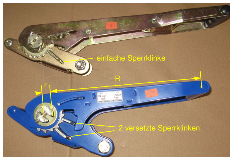
Bild 7: Spannratschen
