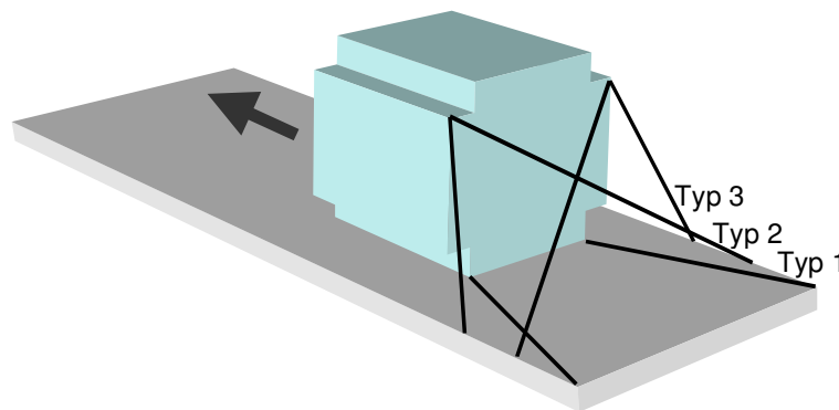
Bild 37: Komplexe Direktzurrung
