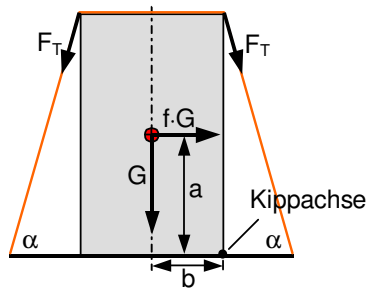
Bild 2: Traditionelle Bewertung einer Niederzurrung
