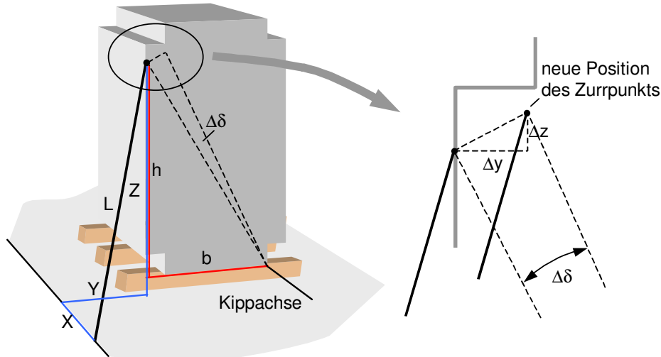
Bild 34: Direktsicherung gegen Kippen
