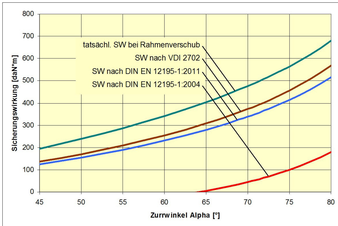
Bild 22: Sicherungswirkung Momente quer, Vergleich von Rechenmodellen
