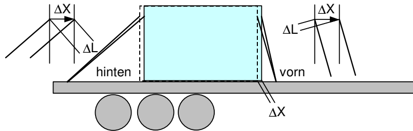
Bild 35: Asymmetrische Direktzurrung
