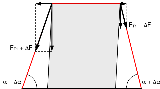
Bild 17: Sicherungswirkung durch Kräfte quer zum Fahrzeug
