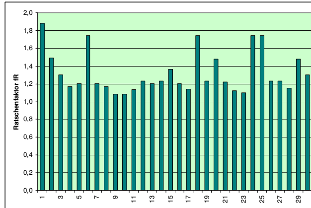
Bild 10: Ratschenfaktoren einer zufälligen Stichprobe bei 2 m Gurtabschnittlänge
