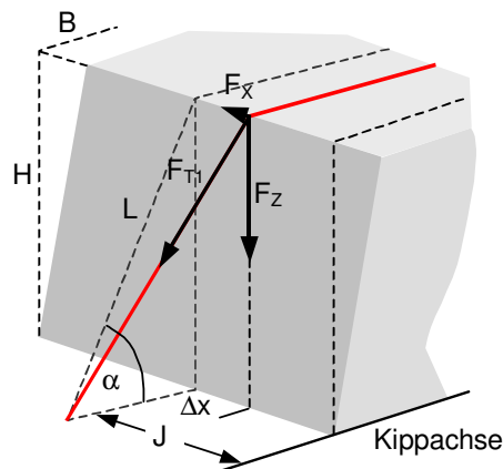
Bild 23: Sicherungswirkung durch Momente längs zum Fahrzeug
