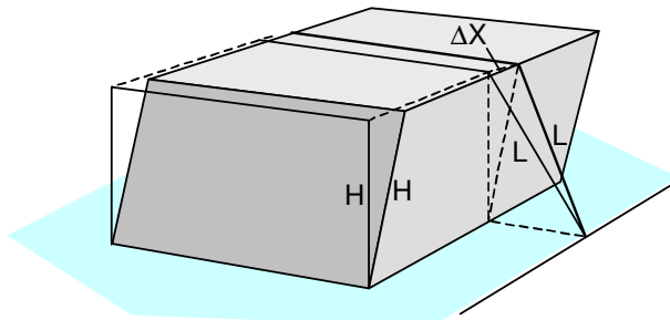
Bild 15: \Delta L bei Rahmenverschub längs zum Fahrzeug
