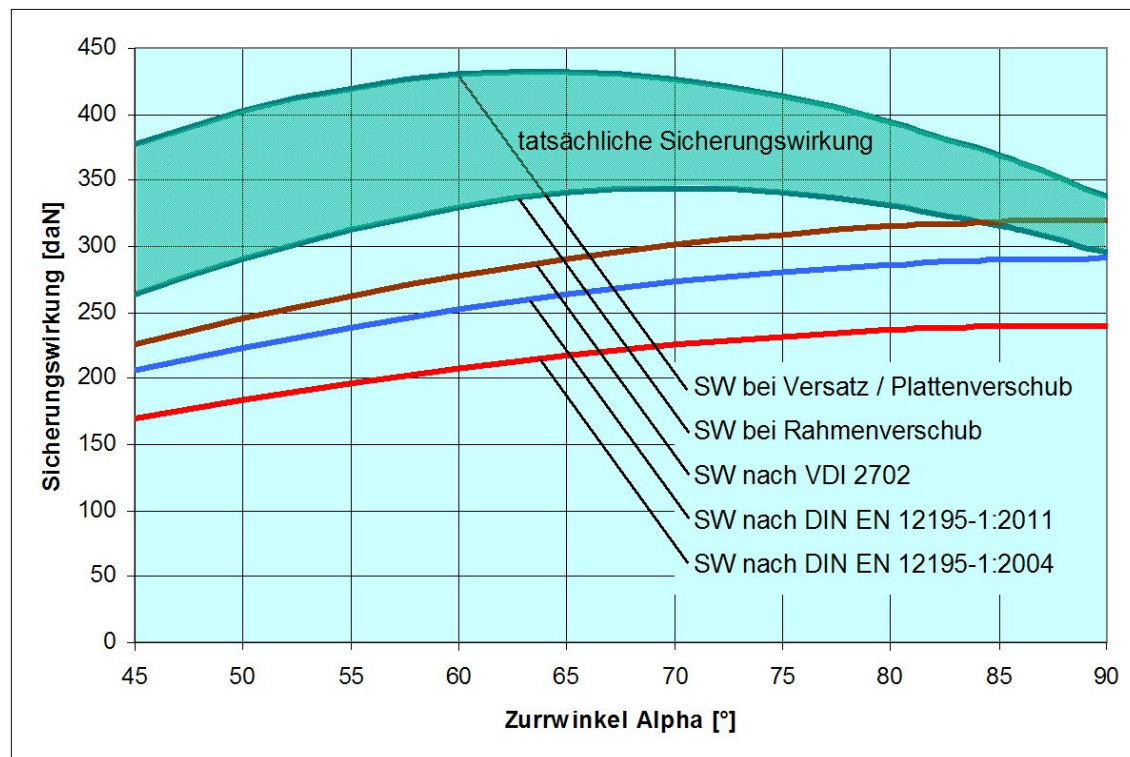
Bild 18: Sicherungswirkung Kräfte quer, Vergleich von Rechenmodellen
