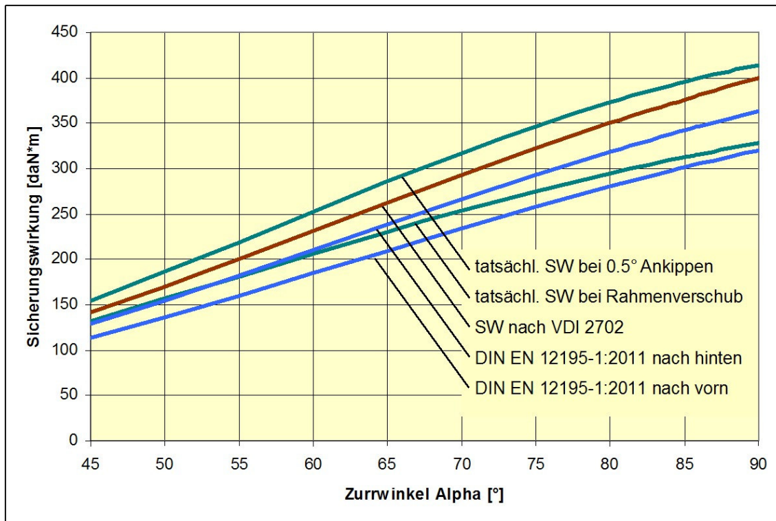
Bild 24: Sicherungswirkung Momente längs, Vergleich von Rechenmodellen
