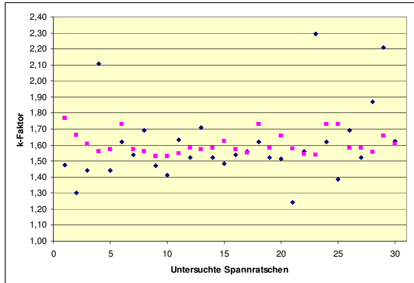
Bild 8: k'-Faktoren von Spannratschen
