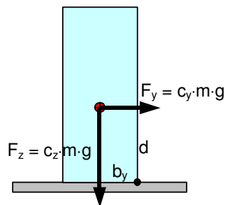
Bild 41: Kippsicherheit durch Eigenstandfestigkeit
