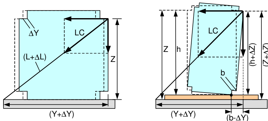
Bild 36: Sicherungswirkungen gegen Rutschen und Kippen
