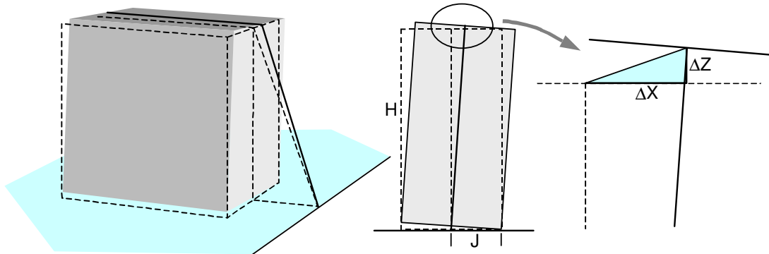
Bild 16: \Delta L beim Ankippen längs zum Fahrzeug
