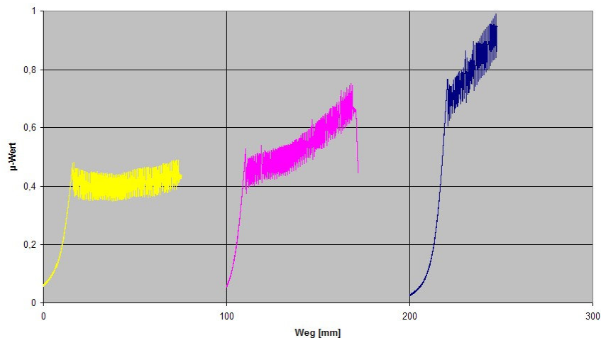
Bild 32: Reibbeiwerte im Zugversuch mit Niederzurrung (Quelle: Flog)
