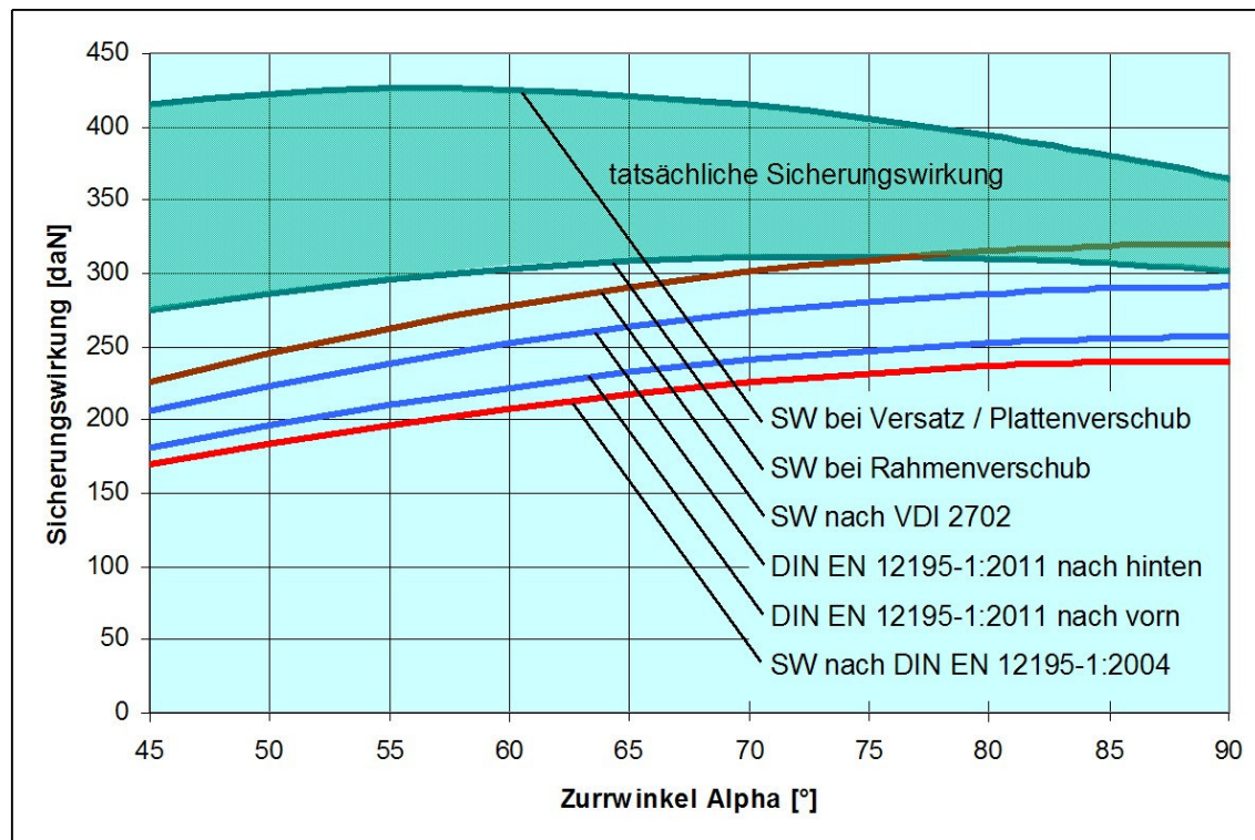
Bild 20: Sicherungswirkung Kräfte längs, Vergleich von Rechenmodellen
