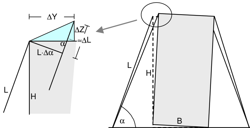
Bild 13: \Delta\alpha und \Delta L links beim Ankippen quer zum Fahrzeug
