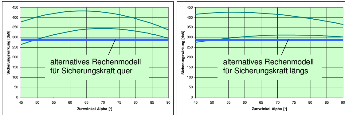
Bild 29: Alternatives Modell der Sicherungswirkung (blau)
