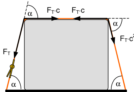
Bild 5: Vorspannungsverlust durch Reibung an den Ladungskanten
