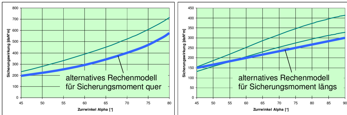
Bild 30: Alternative Modelle der Sicherungswirkung (blau)
