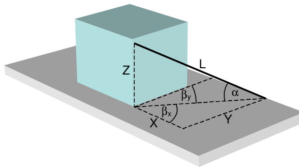
Bild 33: Geometrie einer Direktzurrung
