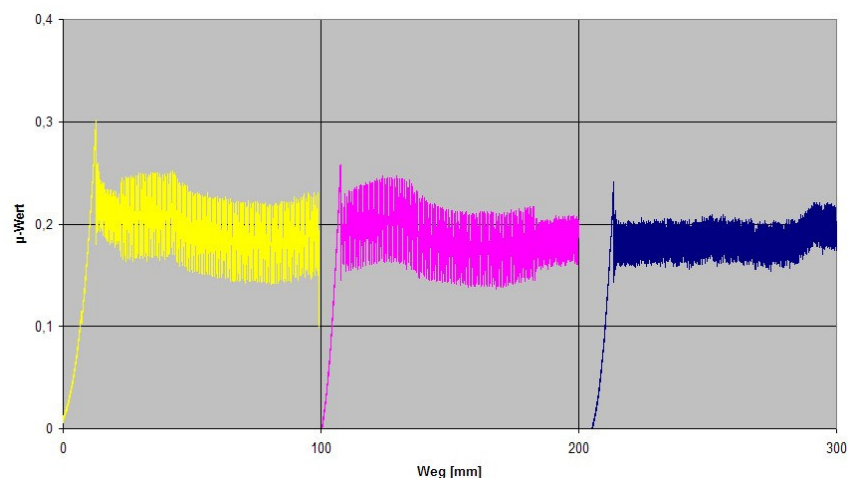
Bild 31: Reibbeiwerte im Zugversuch ohne Niederzurrung (Quelle: Flog)
